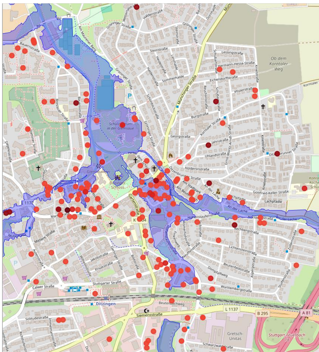
Abbildung 26: Starkregenereignisse von 2010
