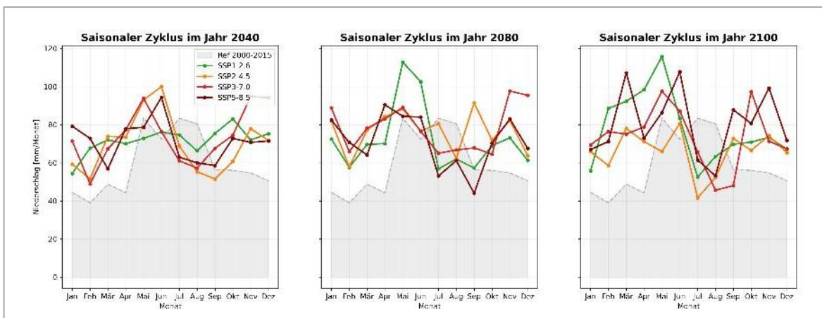
Abbildung 12: Saisonaler Zyklus der Niederschläge
