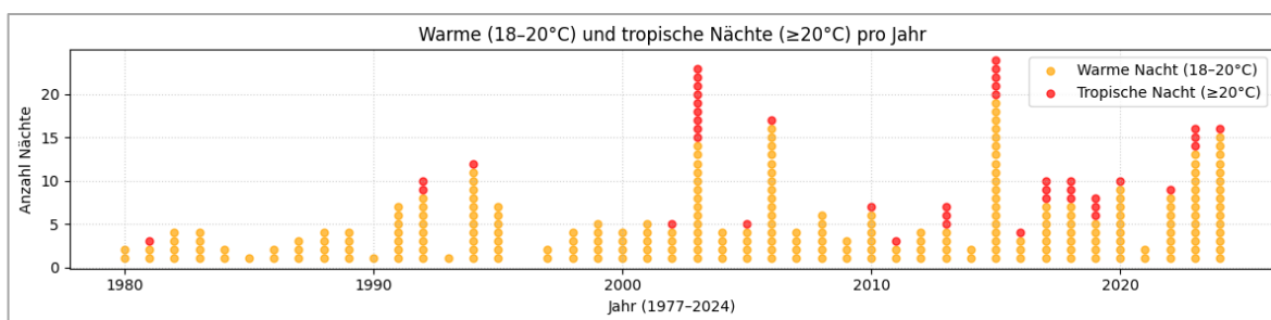
Abbildung 8: Warme Nächte und Tropennächte pro Jahr
