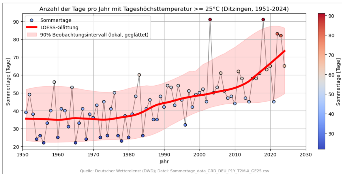
Abbildung 6: Sommerstage pro Jahr
