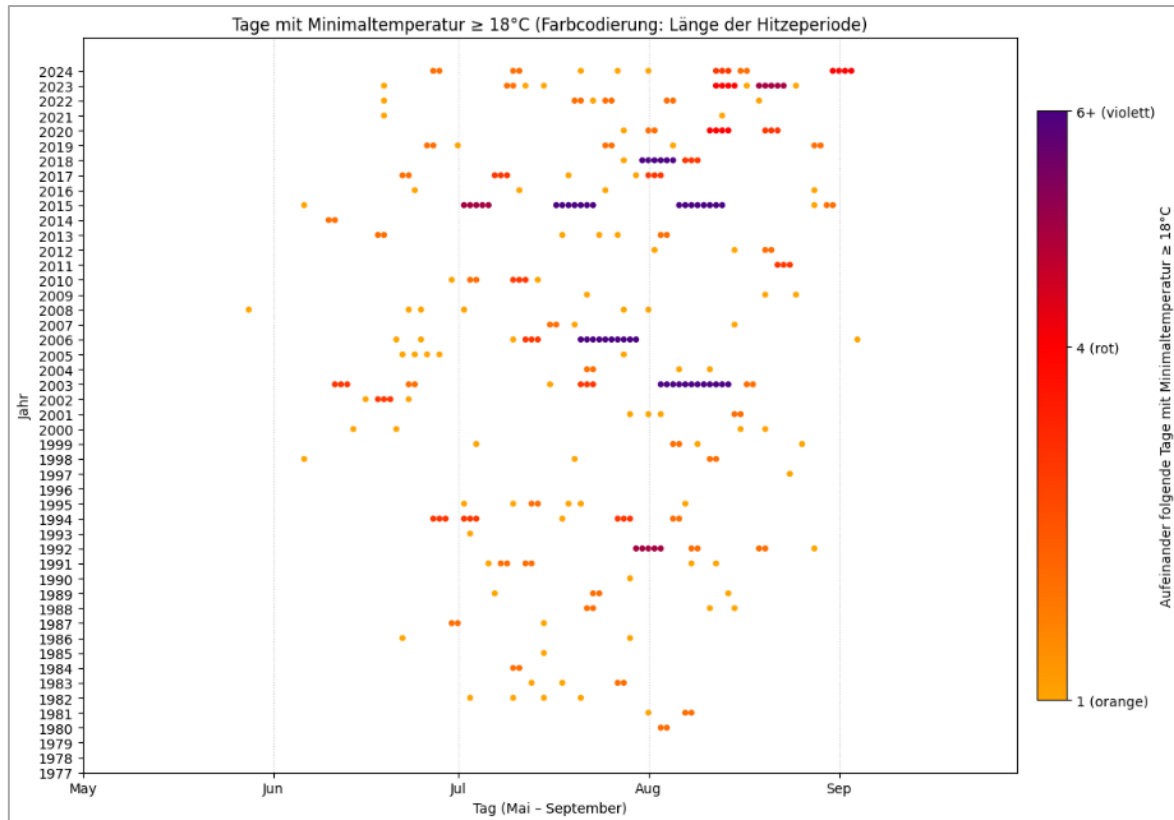
Abbildung 10: Warme Nächte in Folge
