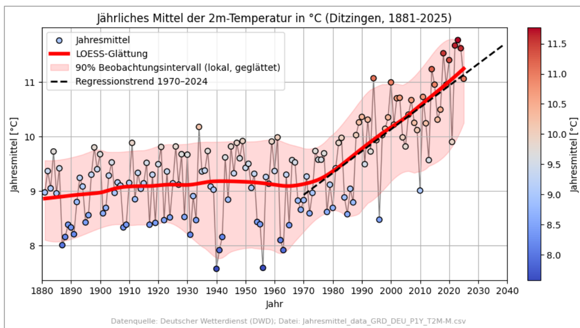
Abbildung 4: Jahresmittel Ditzingen
