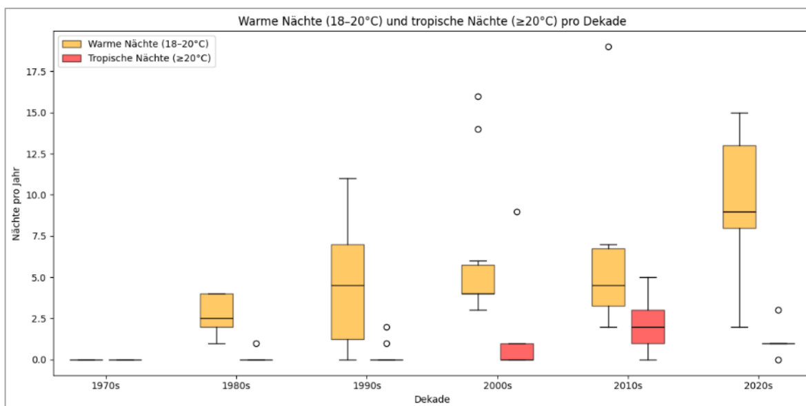
Abbildung 9: Warme Nächte und Tropennächte pro Dekade
