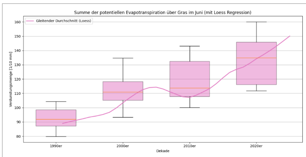
Abbildung 16: Verdunstung im Juni in Ditzingen
