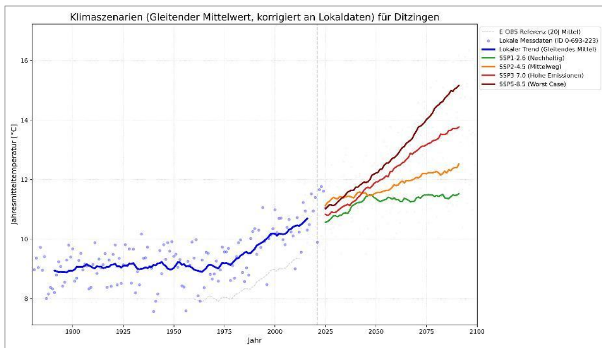
Abbildung 5: Klimaszenarien für Ditzingen
