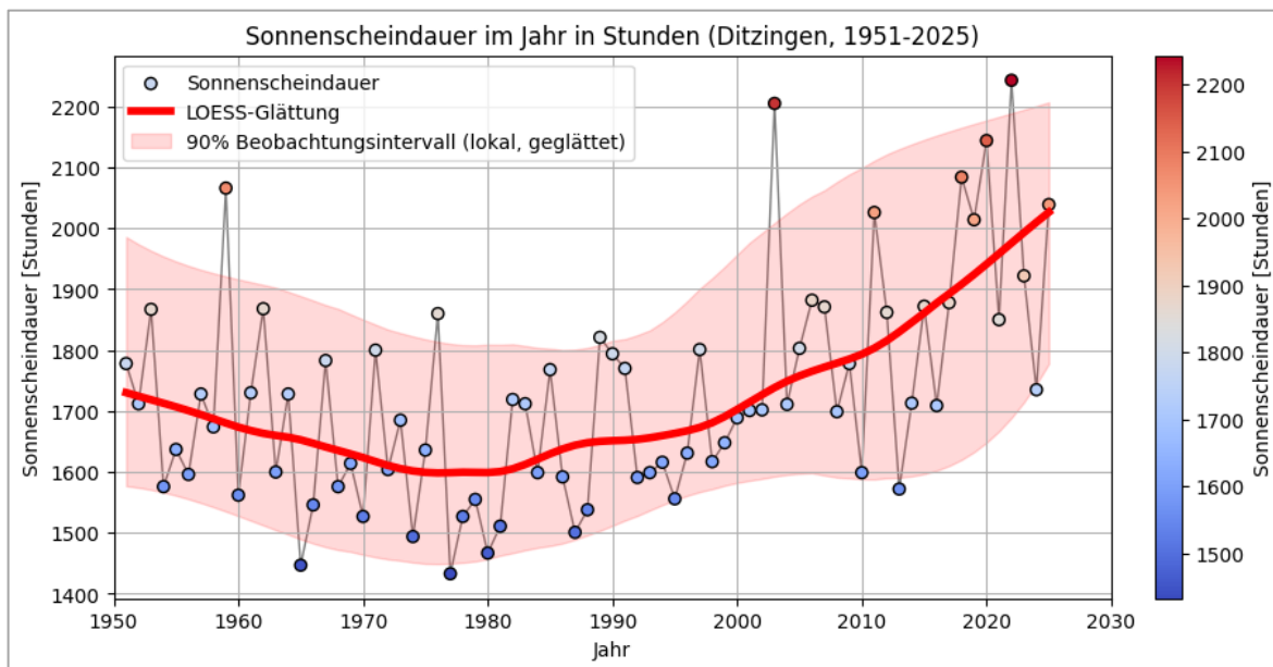
Abbildung 11: Jährliche Sonnenscheindauer
