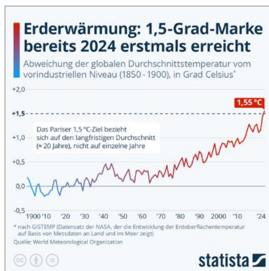
Abbildung 34: Globale Temperaturzunahme
