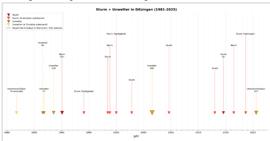
Abbildung 18: Unwetter und Stürme in Ditzingen
