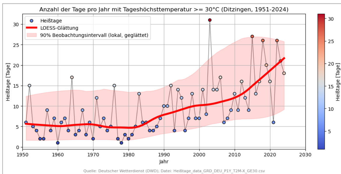
Abbildung 7: Heißtage pro Jahr
